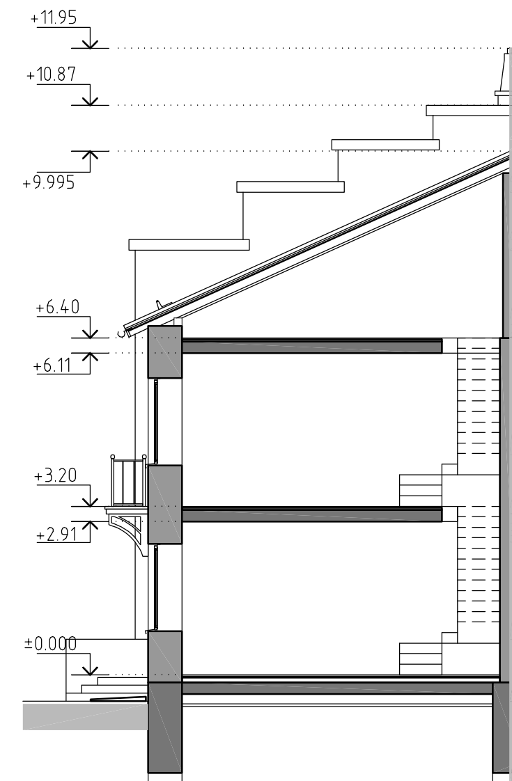
РАЗРЕЗ 1-1
