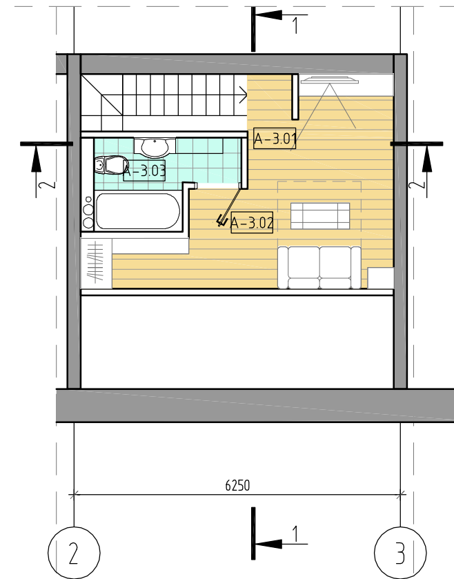
Мансардный этаж
