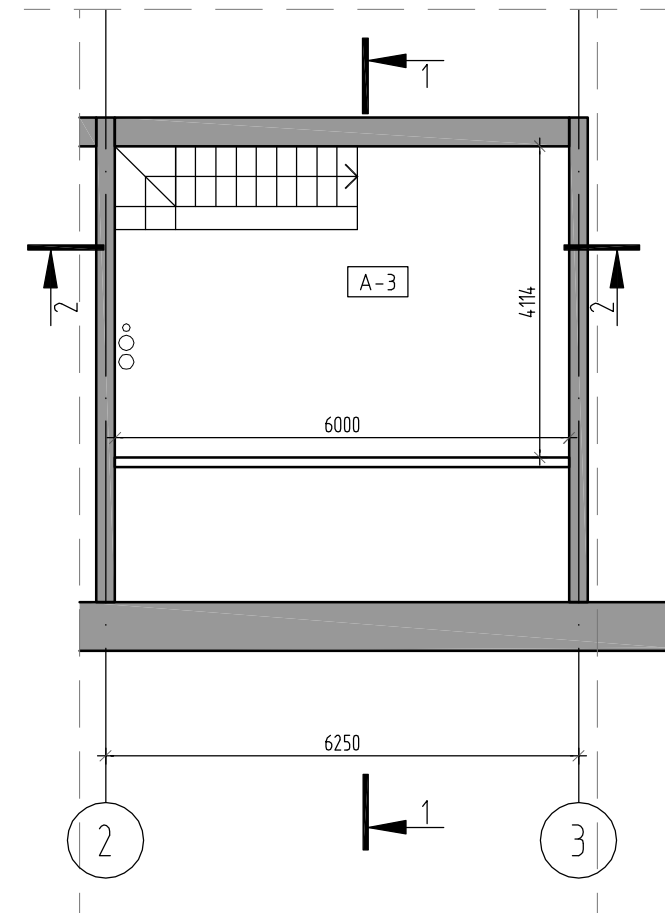
Мансардный этаж
