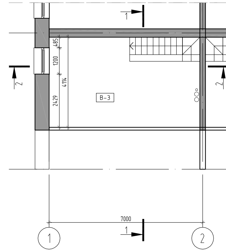
Мансардный этаж
