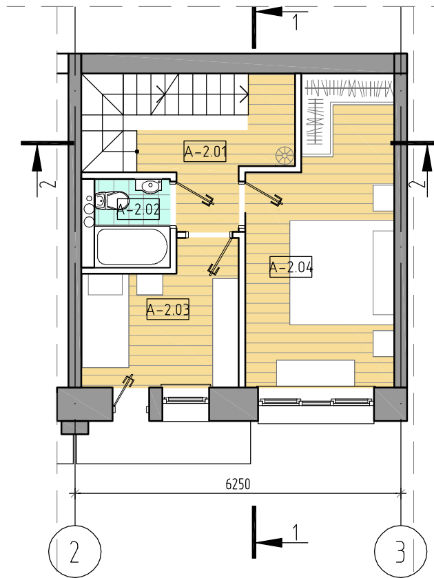
2-этаж
