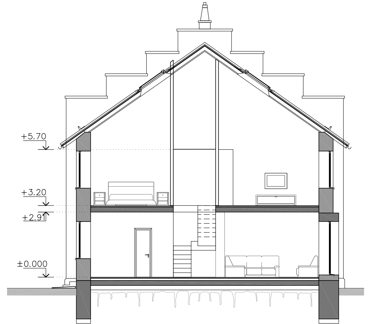
Разрез 1-1
