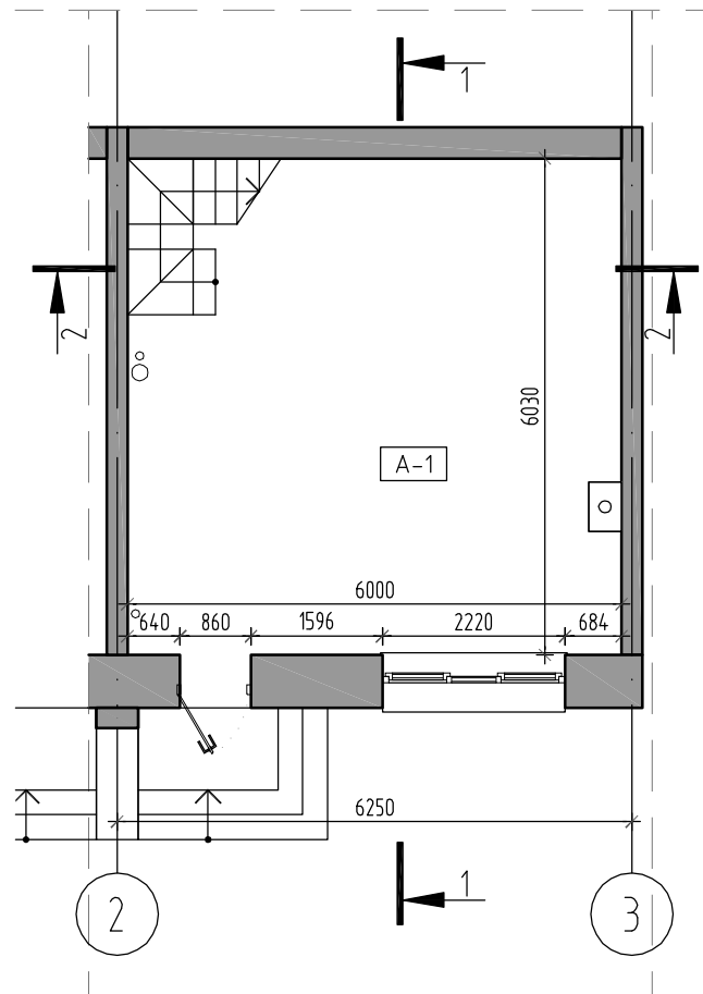
1-этаж
