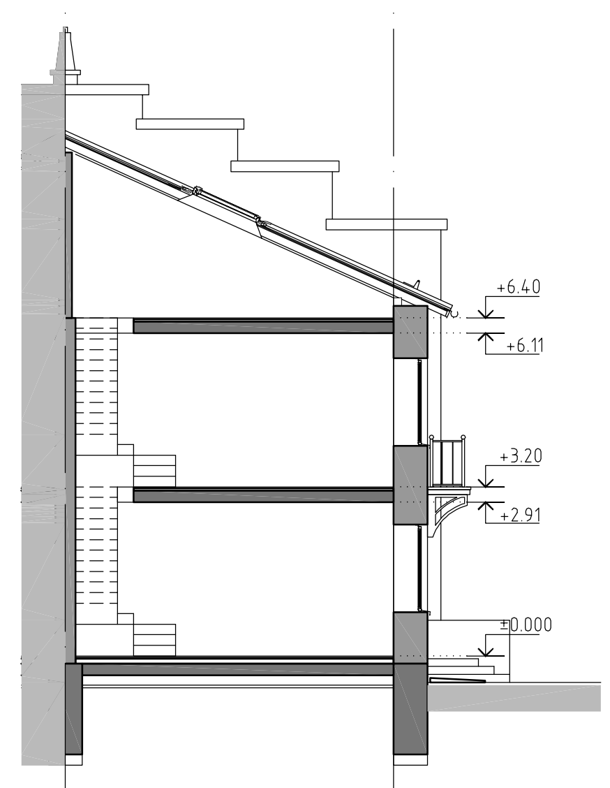
Разрез 1-1
