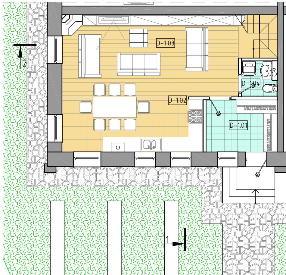
1-этаж
