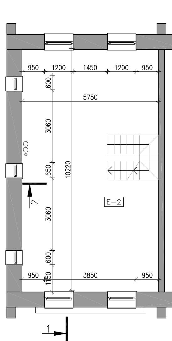
2-этаж
