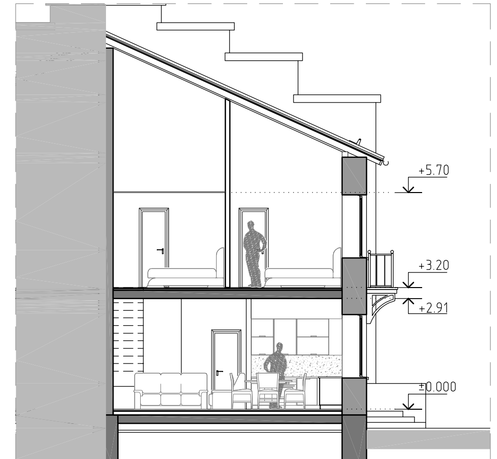
Разрез 1-1
