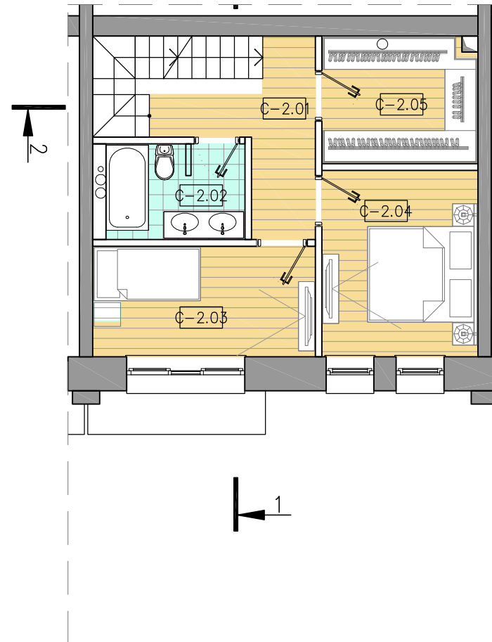
2-этаж
