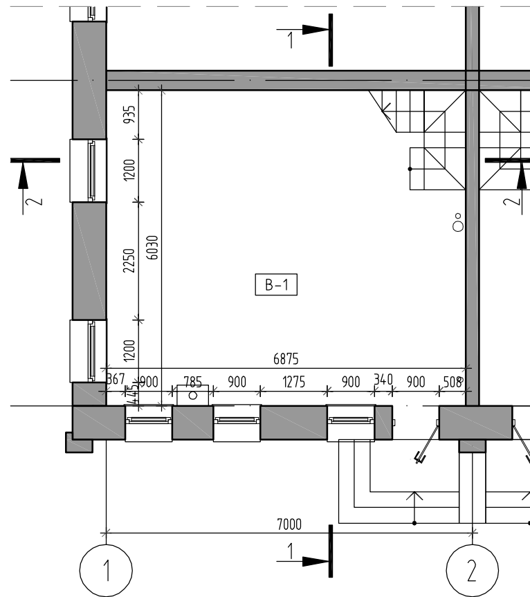
1-этаж
