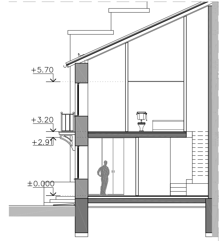
Разрез 1-1
