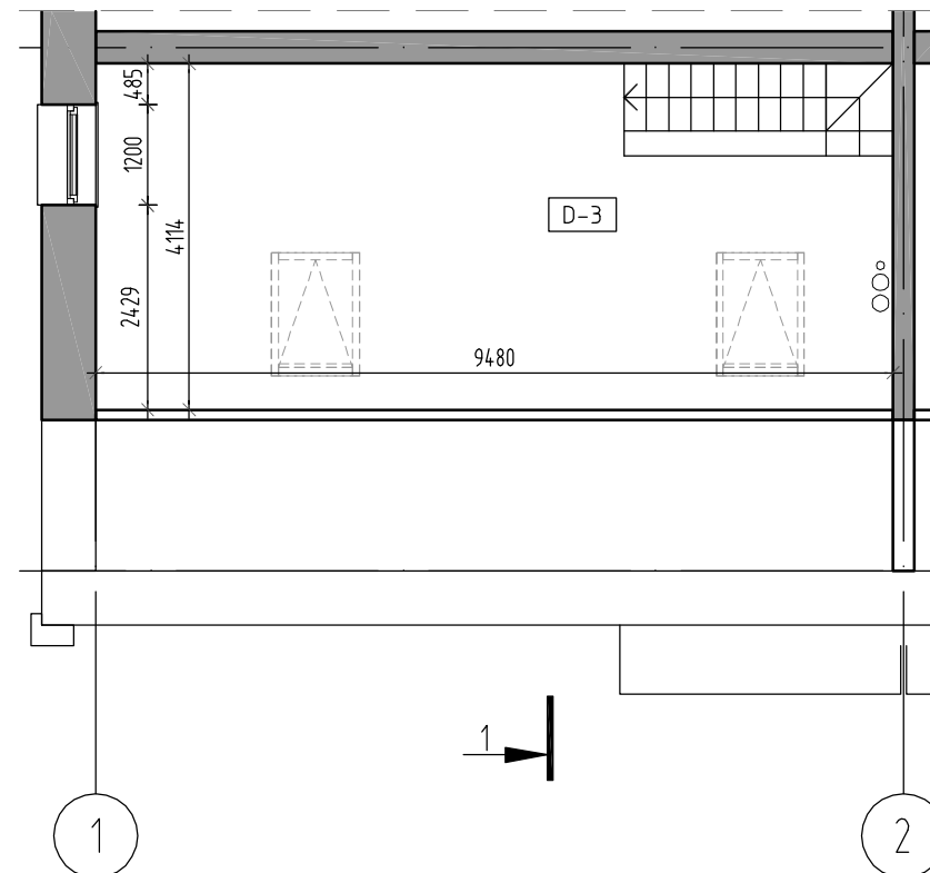
Мансардный этаж
