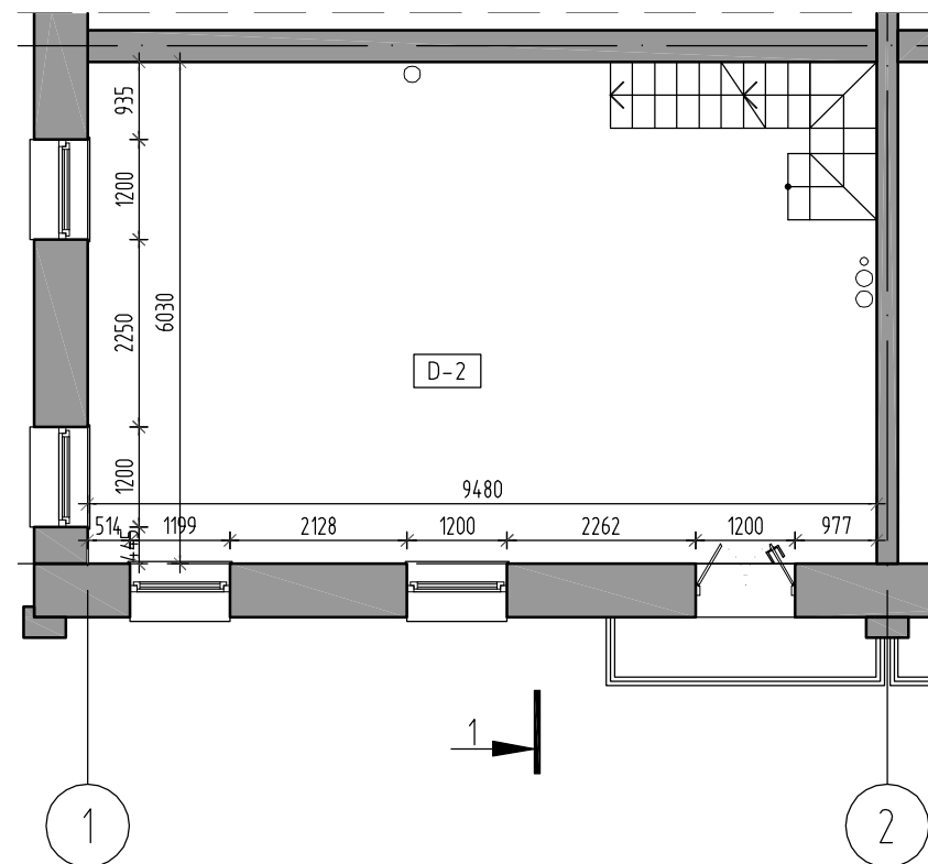
2-этаж
