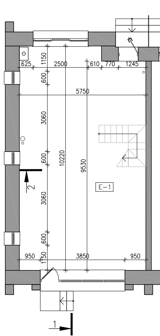
1-этаж
