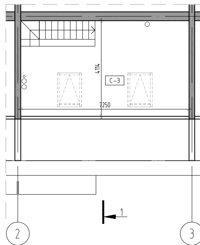
Мансардный этаж
