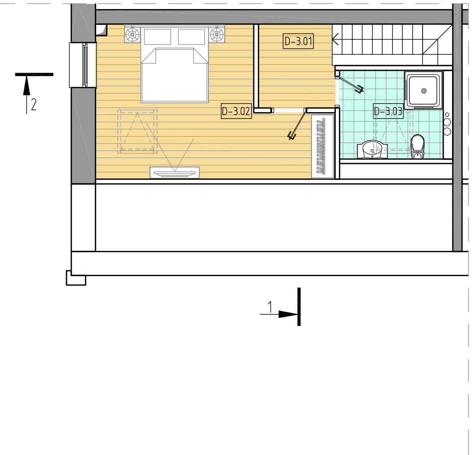
Мансардный этаж
