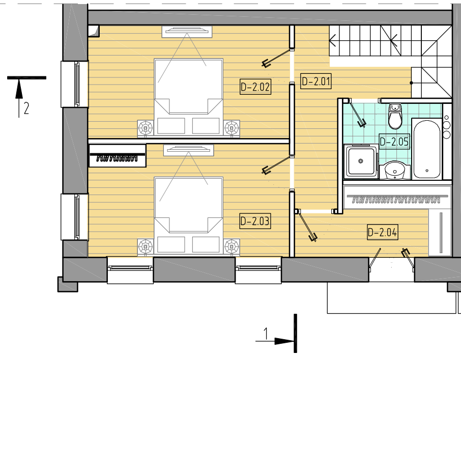
2-этаж
