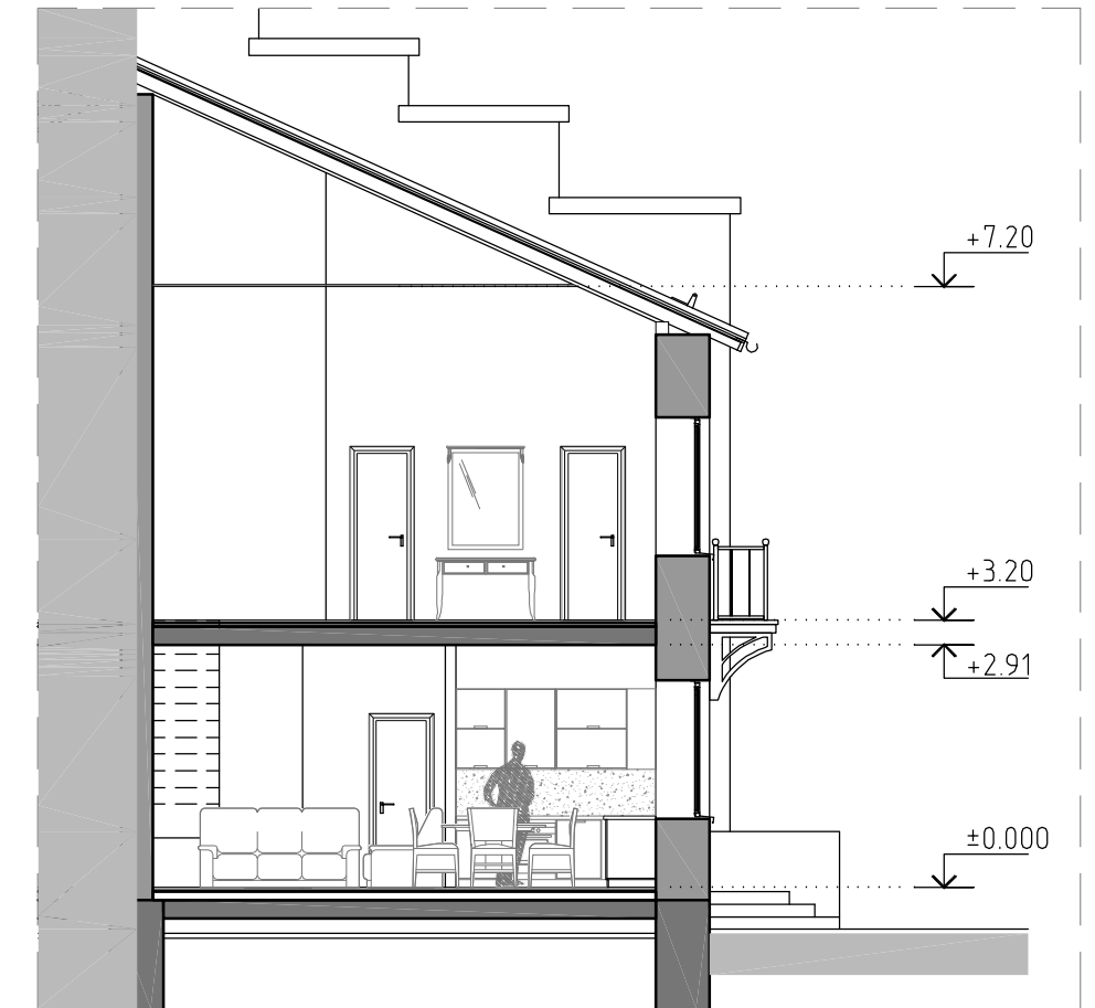
Разрез 1-1
