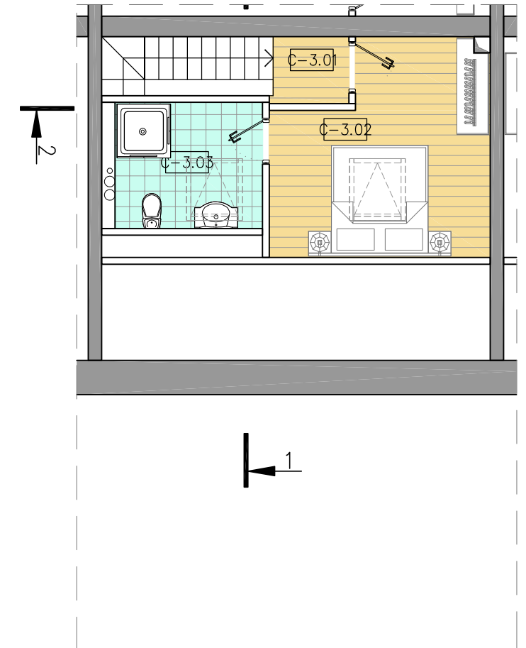
Мансардный этаж
