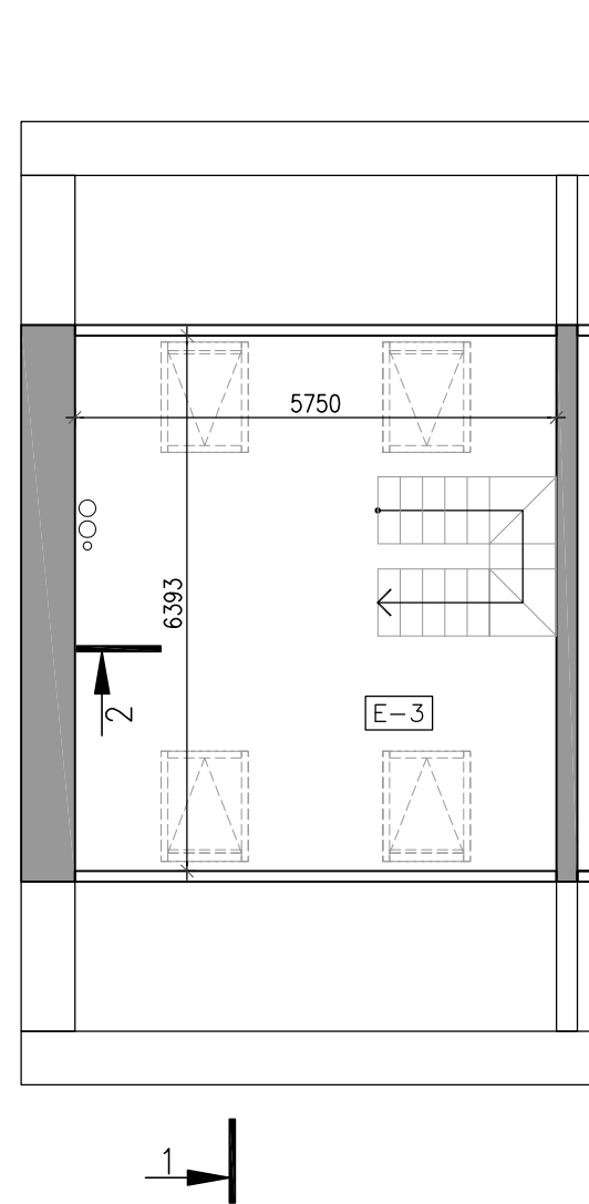
Мансардный этаж
