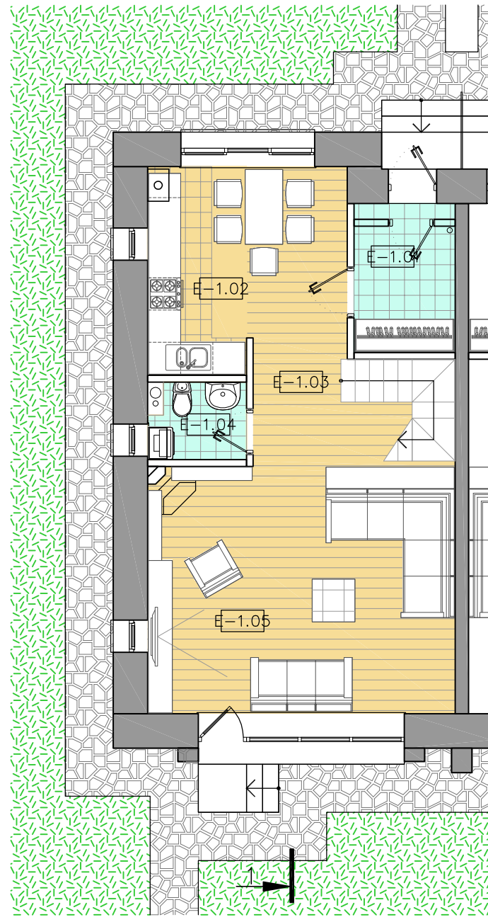
1-этаж
