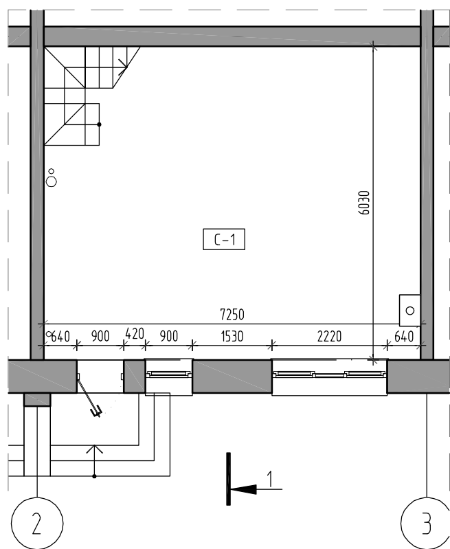
1-этаж
