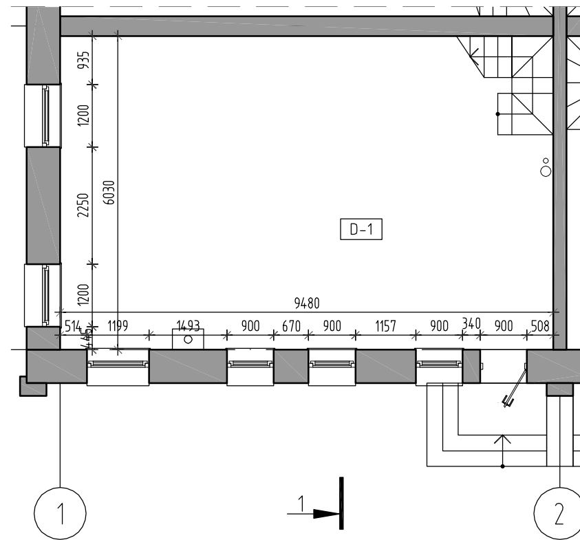
1-этаж
