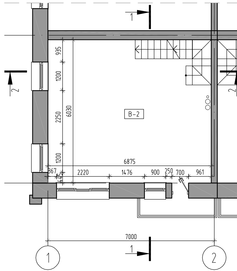
2-этаж
