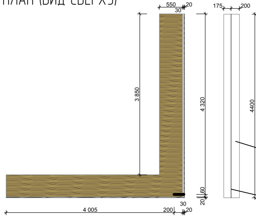
ПЛАН (ВИД СВЕРХУ)
