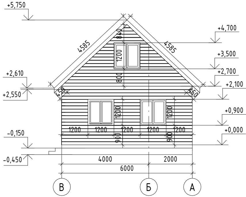
Фасад В-А
