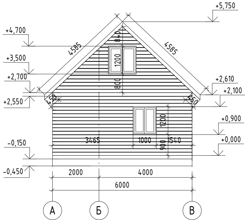
Фасад А-В
