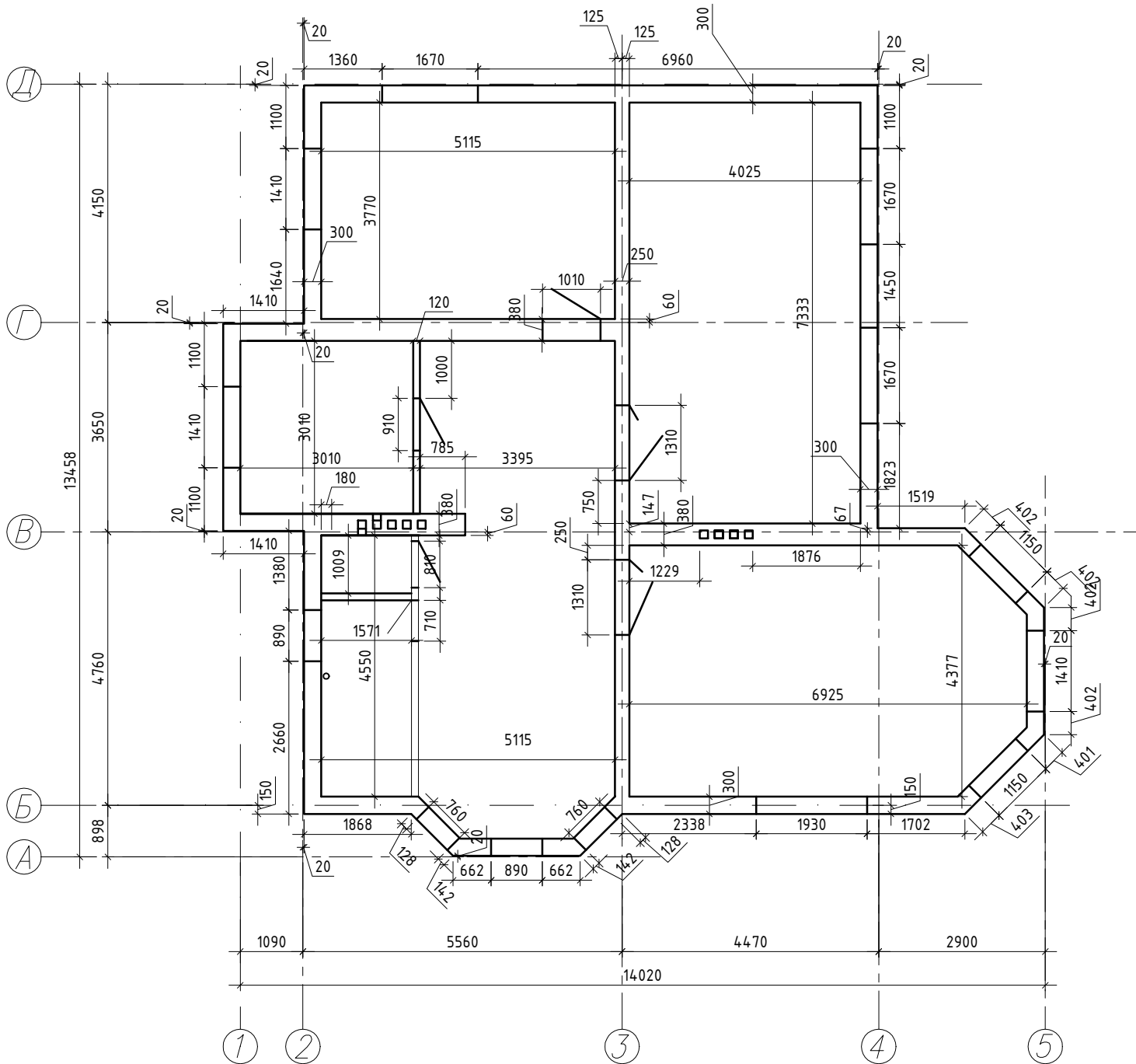
Кладочный план 2-го этажа
