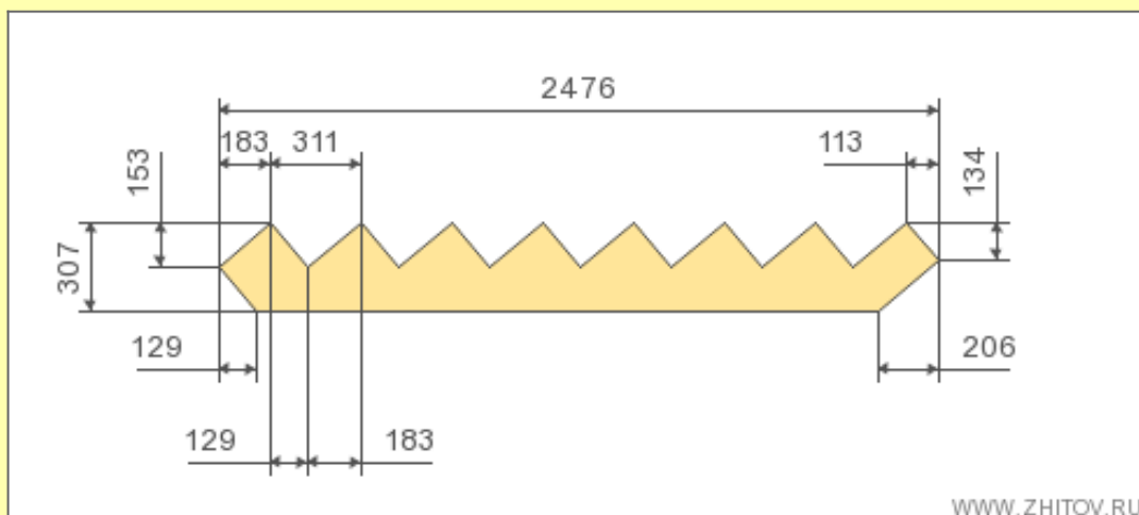
Чертеж косоура
