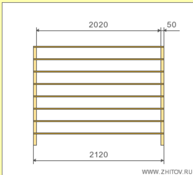
Вид спереди
