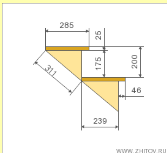
Чертеж ступеней
