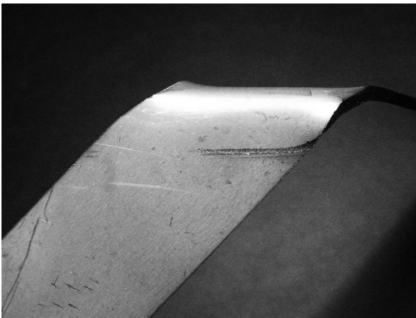
Загибы поверхности от гибки и вмятины от гибочного станка.
