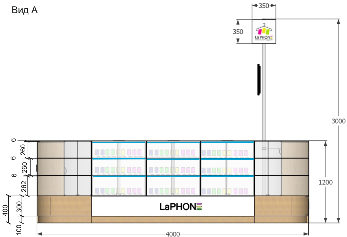
Вид Б
