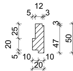
Сечени 1-1
