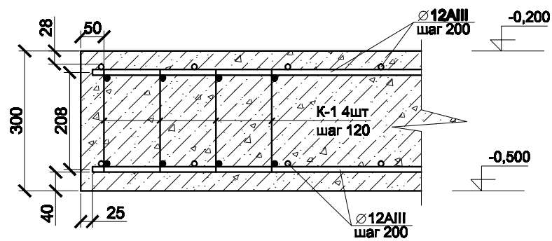
Сечение Б-Б М 1:10
