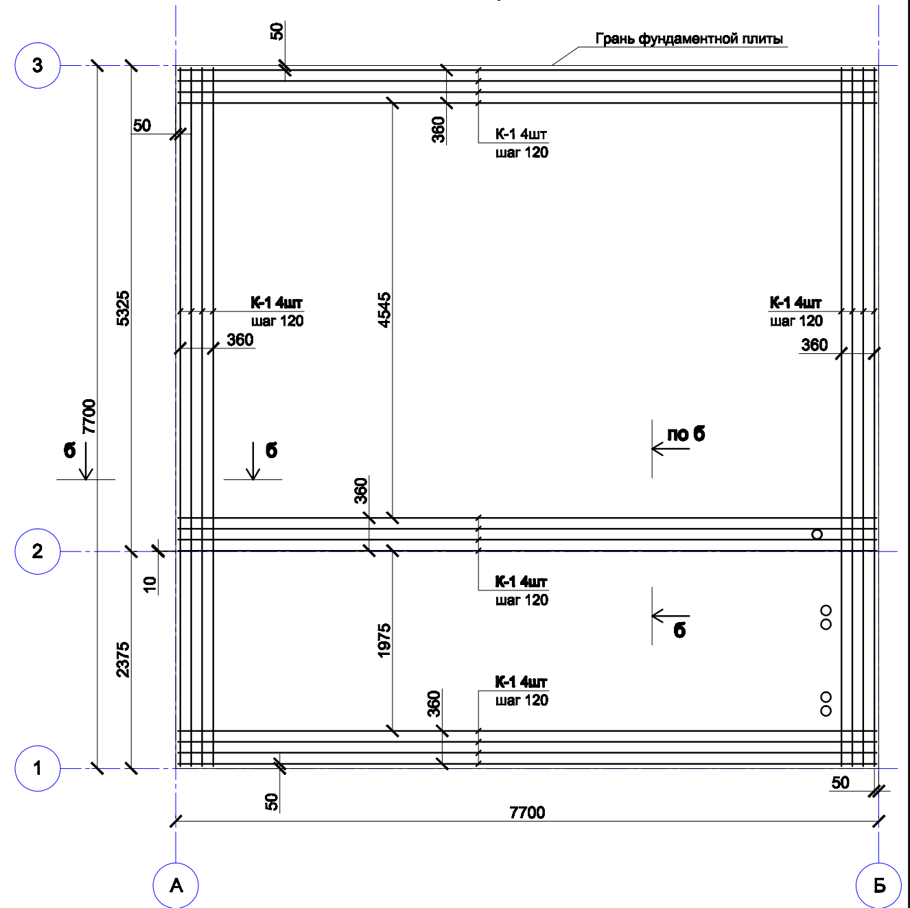
Схема раскладки арматурных каркасов
