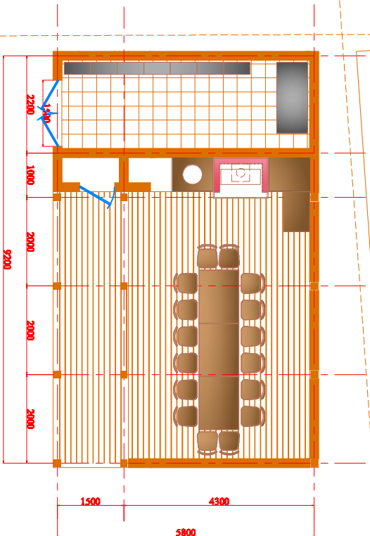
ПЛАН. М 1:100
