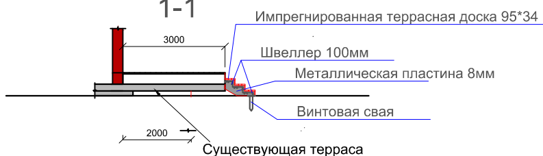
Вариант 2 1-1
