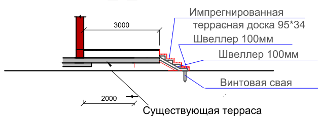
Вариант 1 2-2
