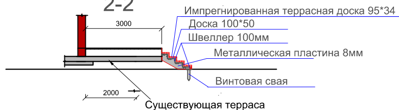
Вариант 2 2-2
