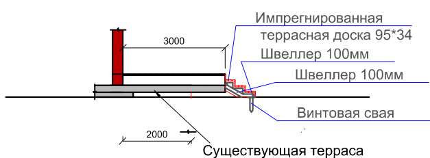
Вариант 1 1-1
