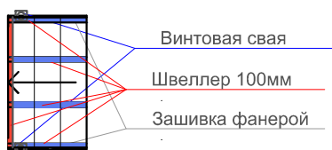
Вариант 1 2-2
