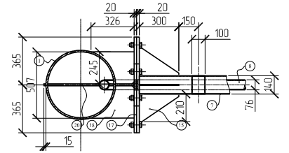
2-2 (М 125)
