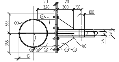
4-4 (М 125)
