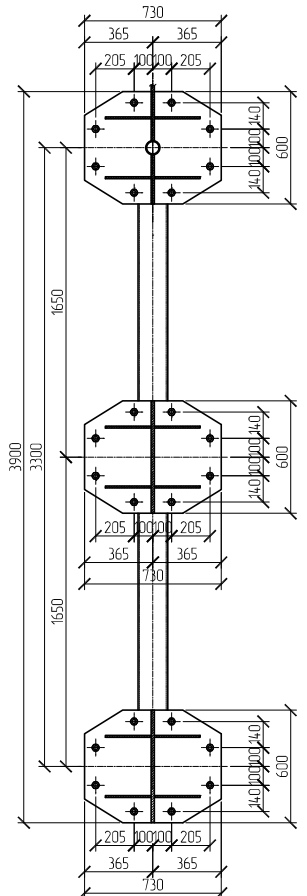
4-4 (М 125)
