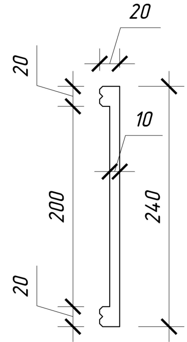
Профиль. Тип 4
