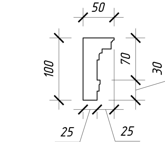
Профиль. Тип 10
