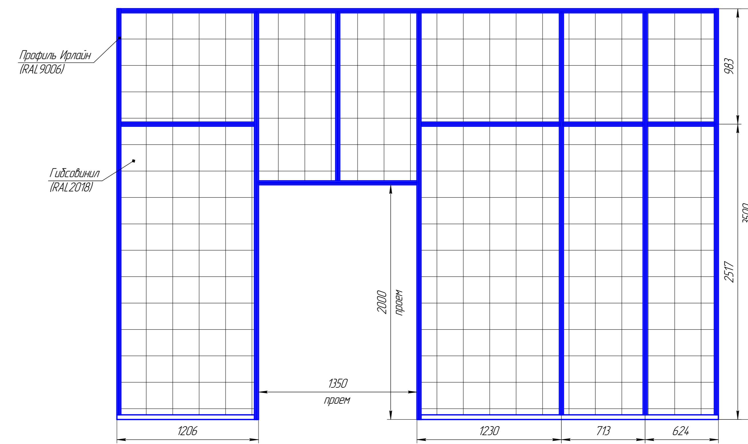
Развертка перегородки "Ирлайн" (вид Б) пом.1
