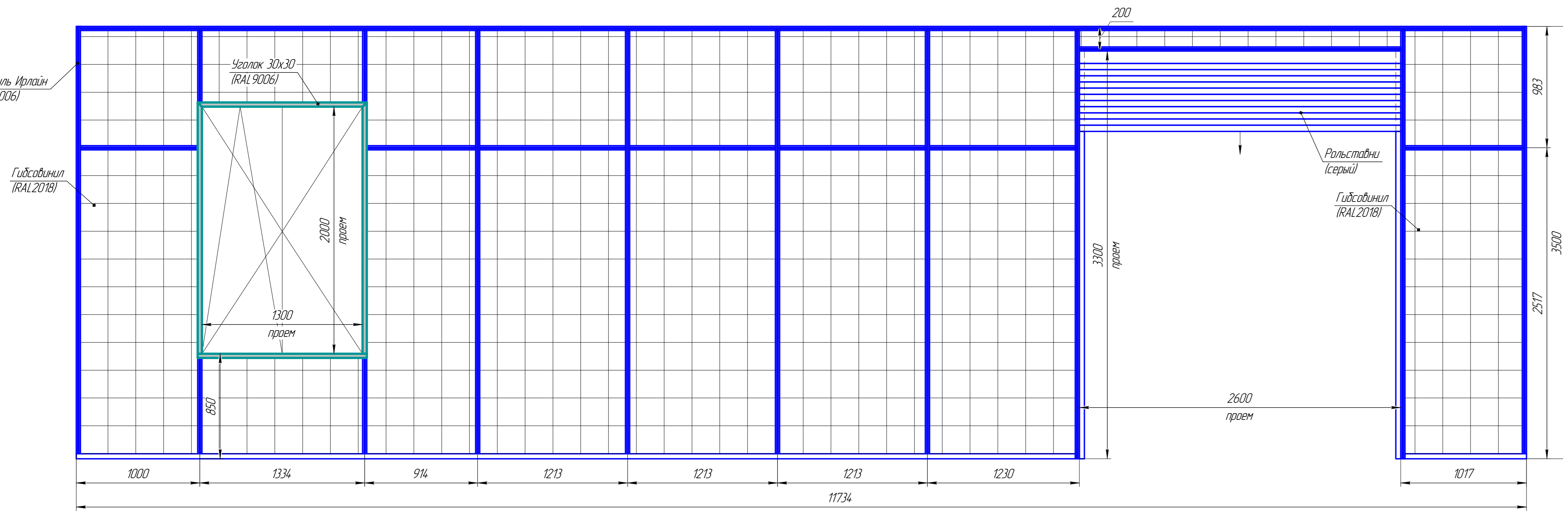
Развертка перегородки "Ирлайн" (вид А) Пом.2
