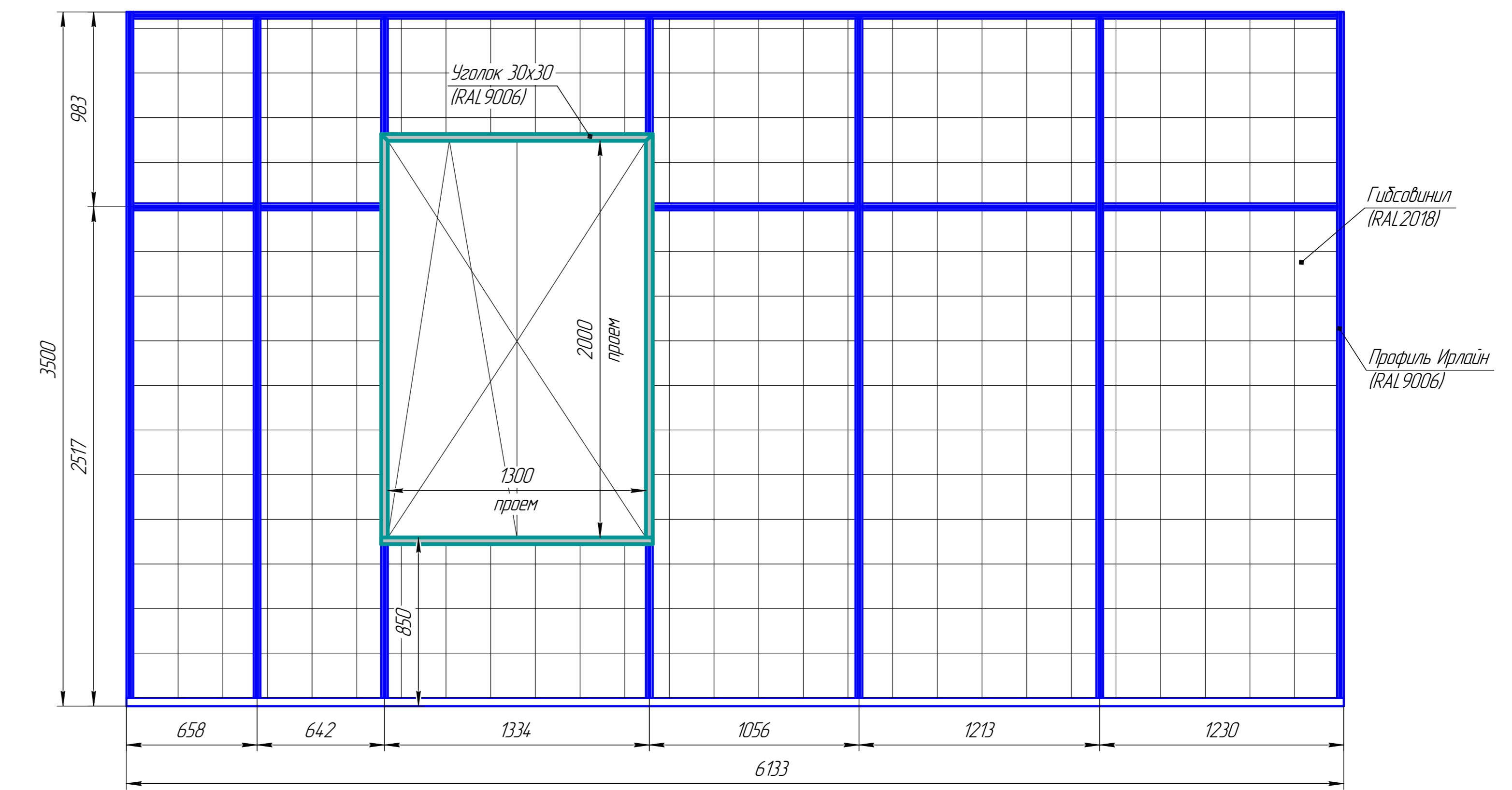
Развертка перегородки "Ирлайн" (вид Е) пом.2
