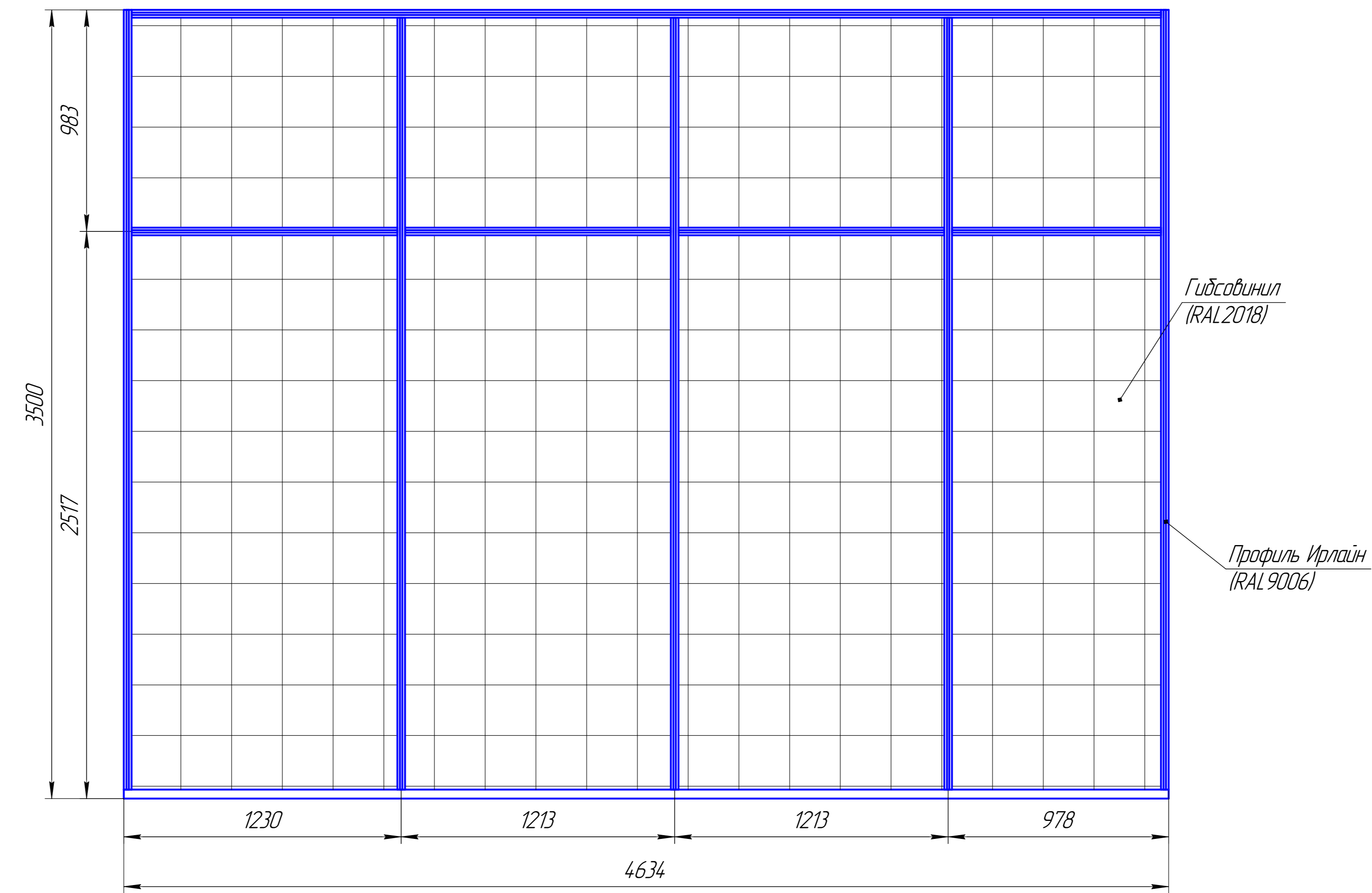
Развертка перегородки "Ирлайн" (вид В) пом.2
