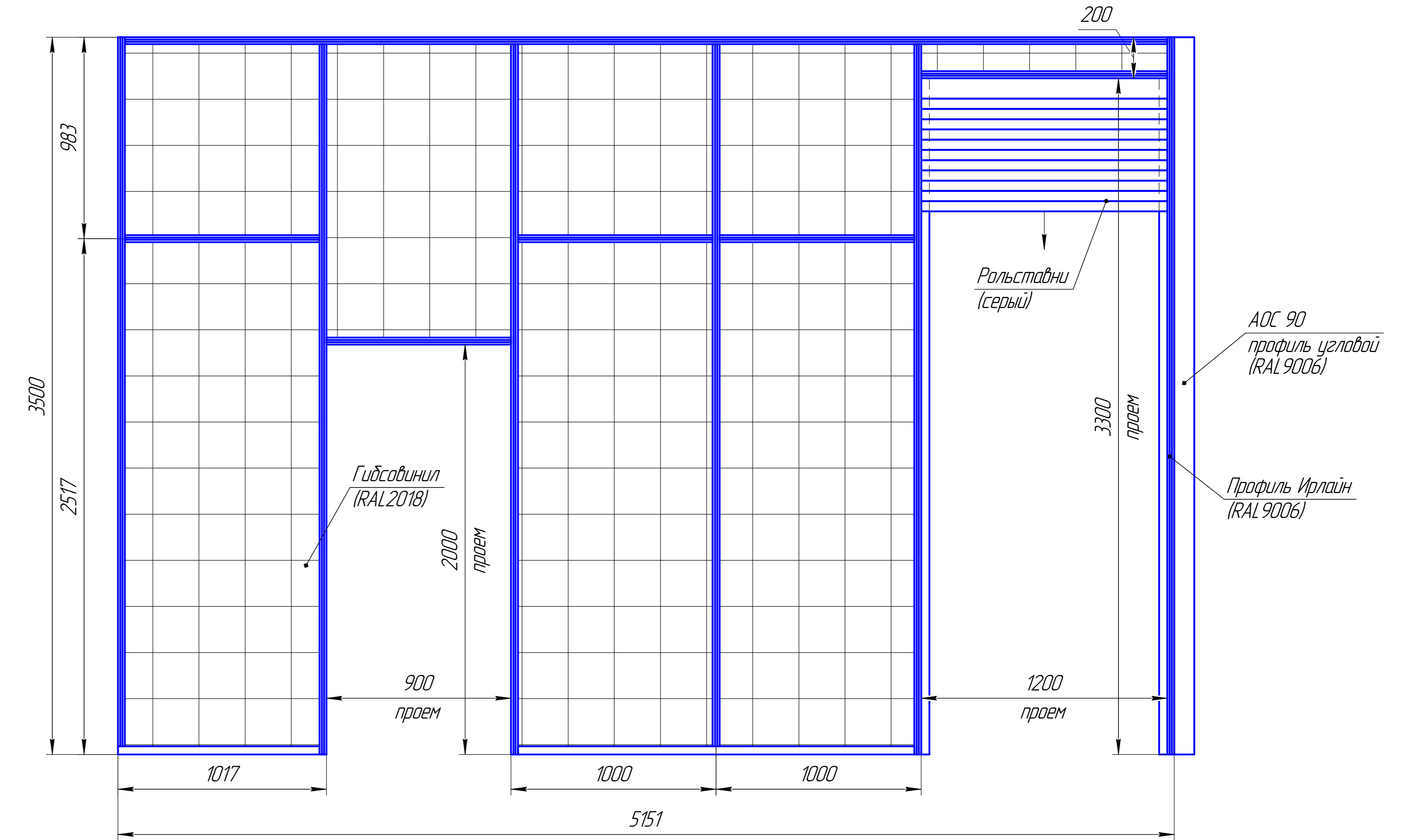
Развертка перегородки "Ирлайн" (вид Г) пом.2
