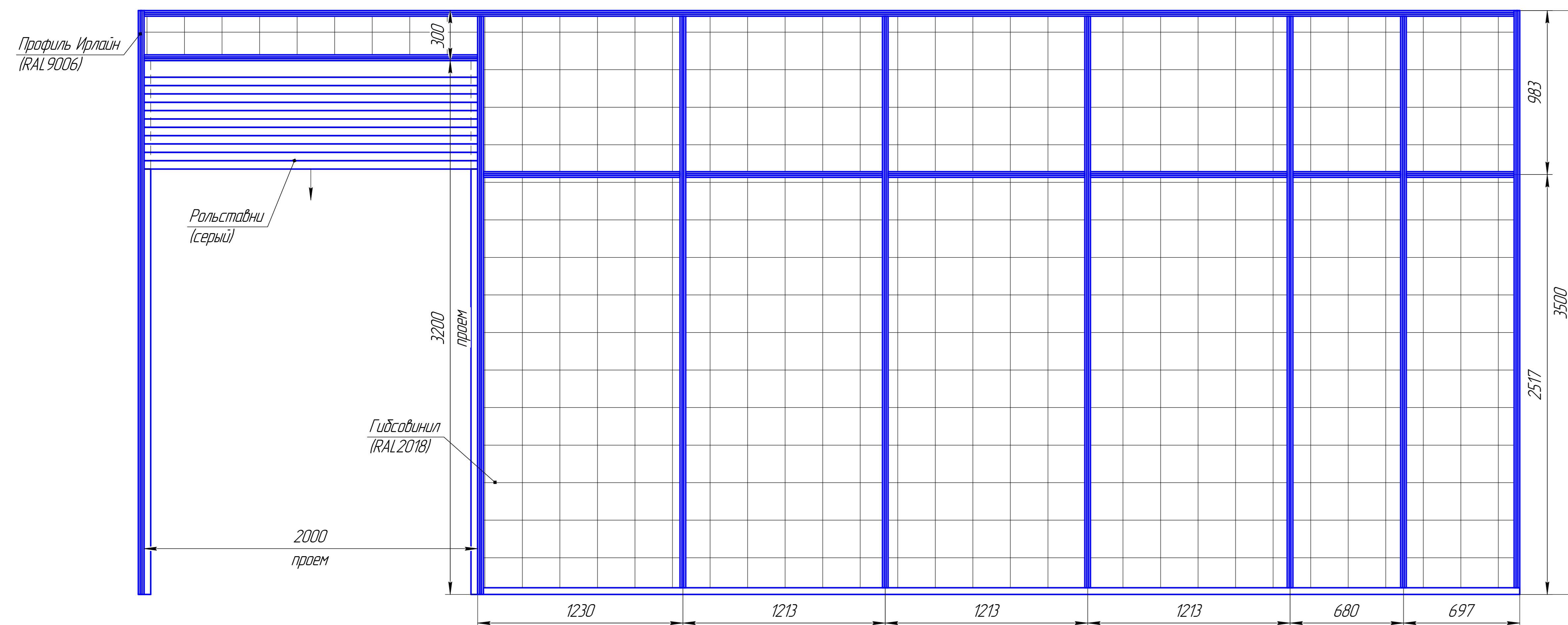
Развертка перегородки "Ирлайн" (вид В) пом.1
