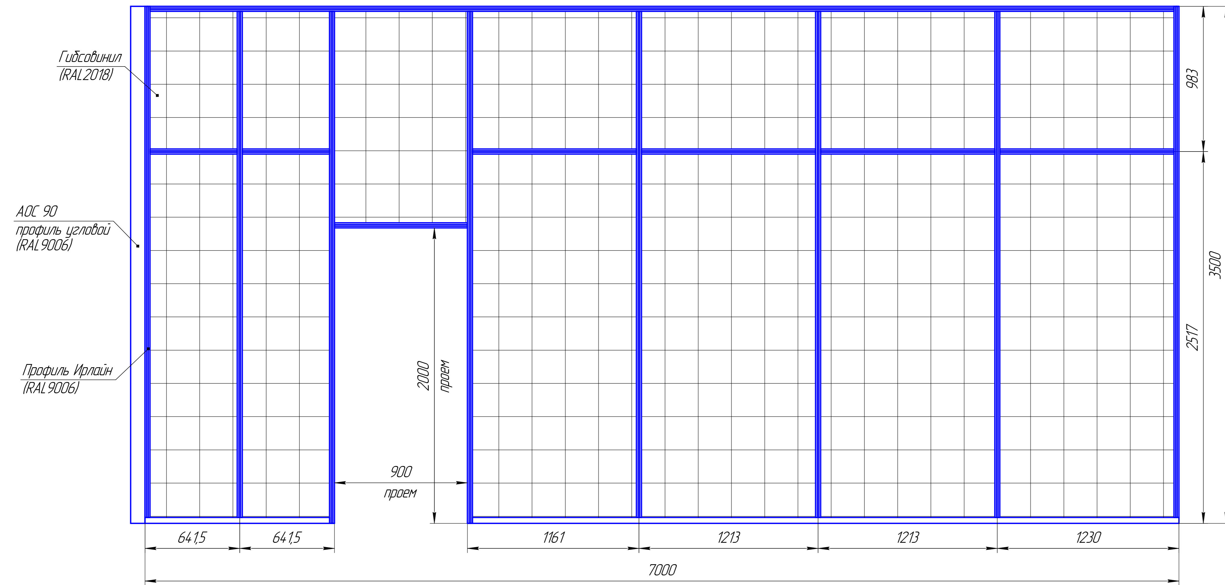
Развертка перегородки "Ирлайн" (вид Д) пом.2
