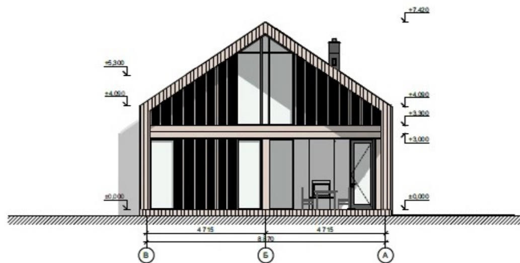
Фасад в осях В - А
