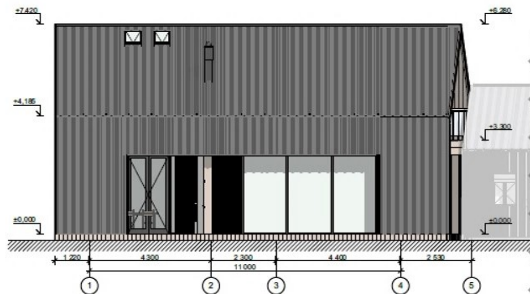
Фасад в осях 1 - 5
