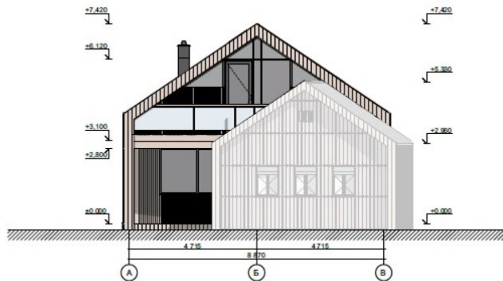
Фасад в осях А - В
