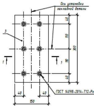
Закладная деталь Мн-1
